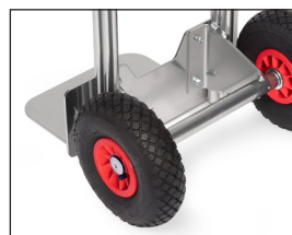
Radbefestigung verschraubte Radbefestigung, einfacher Radwechsel.
