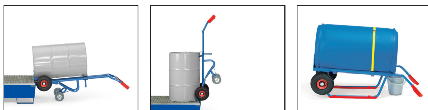
Abstellen eines Fasses auf einer Auffangwanne.
